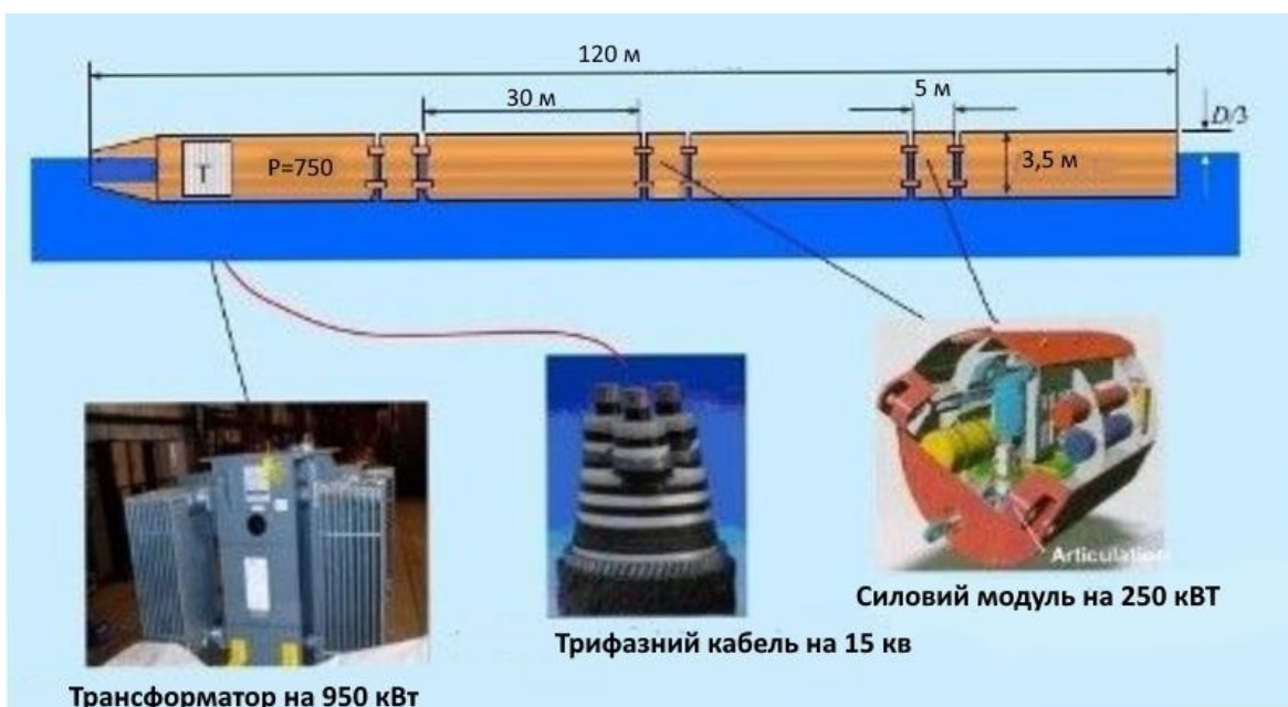
Рис. 1. Pelamis P-750
